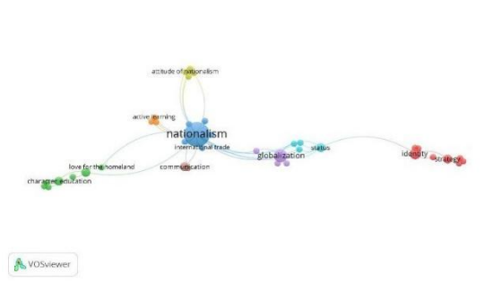
Gambar 3 Network Visualization Kata Kunci Menggunakan VOSviewer
