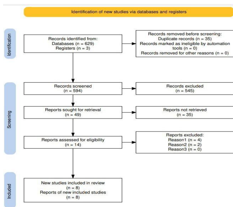
Gambar 2 Diagram Alur Seleksi Artikel Berdasarkan PRISMA 2020
