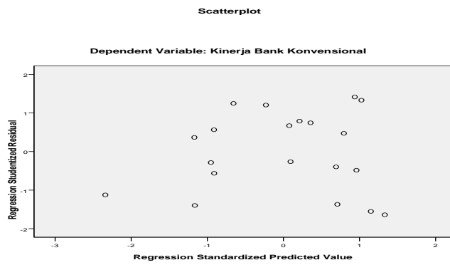
Gambar 3. Scatterplot (BRI)
